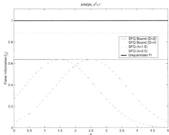
Fig. 3. Parameter in AWGN
